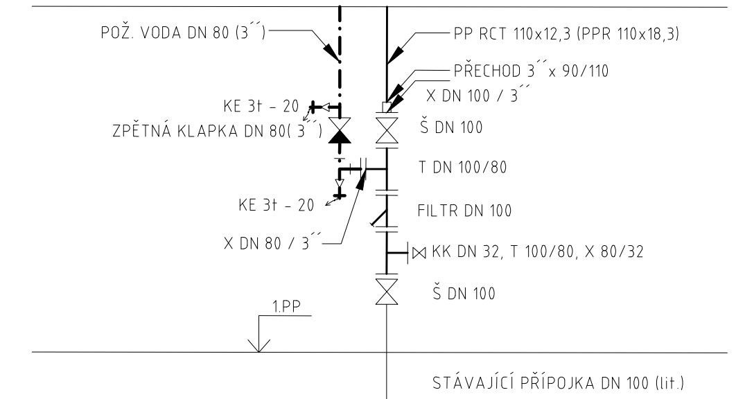
SCHÉMA VSTUPU STUDENÉ A POŽÁRNÍ VODY M 1:50
